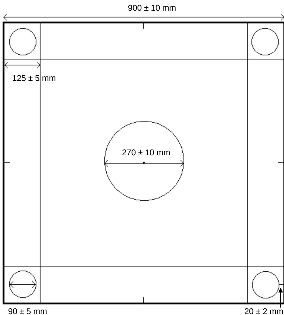
Kuva 1. Kaksinpelissä käytettävän pelipöydän mitat.
