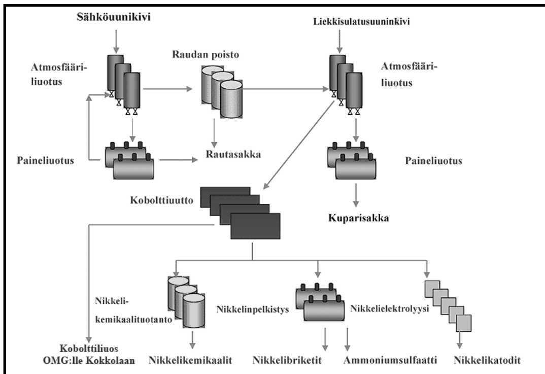
Kuva 1. Norilsk Nickel Hariavalta Oy:n tuotantoprosessin kaaviokuva.
